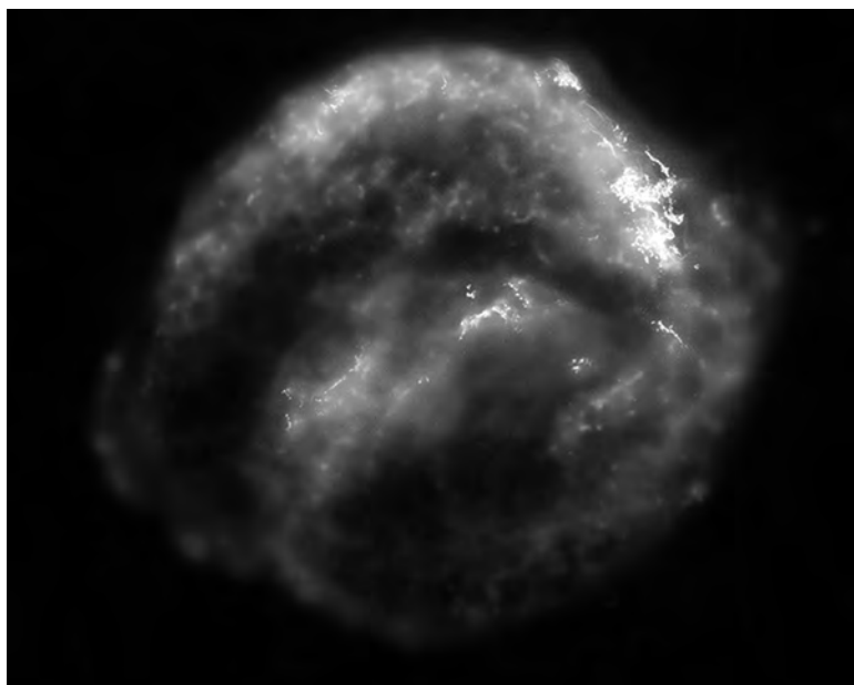
Figura 6. Supernova de Kepler (1604) (NASA/ESA/JHU/R.Sankrit & W. Blair)
