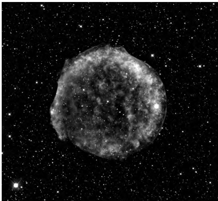
Figura 5. Supernova de 1572 (NASA/MPLA/Calar Alto Observatory, Oliver Krause et ál.)
