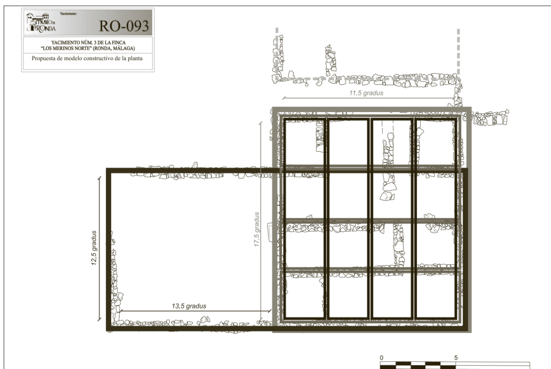
Fig. 7. Propuesta del modelo constructivo
